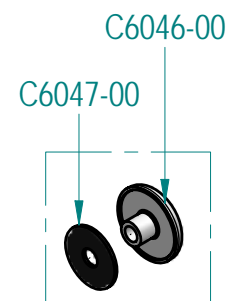
DET. C
