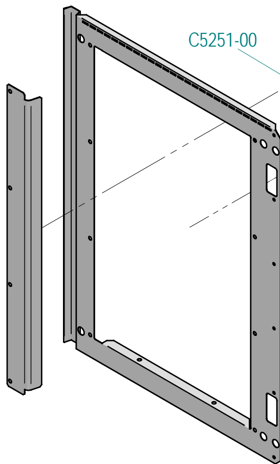
DET. A
