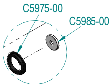
DET. A
