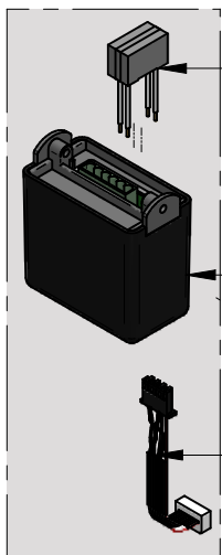
DET. C
