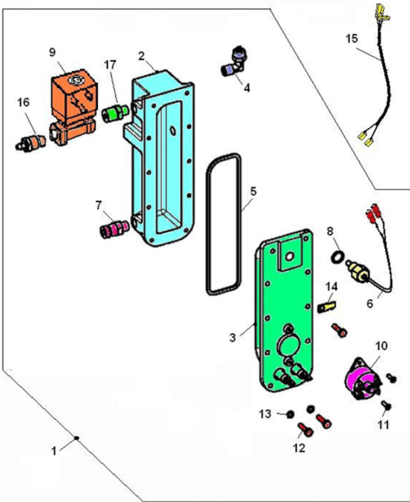
Tavola: C/O ASSIEME CALDAIA (561)
