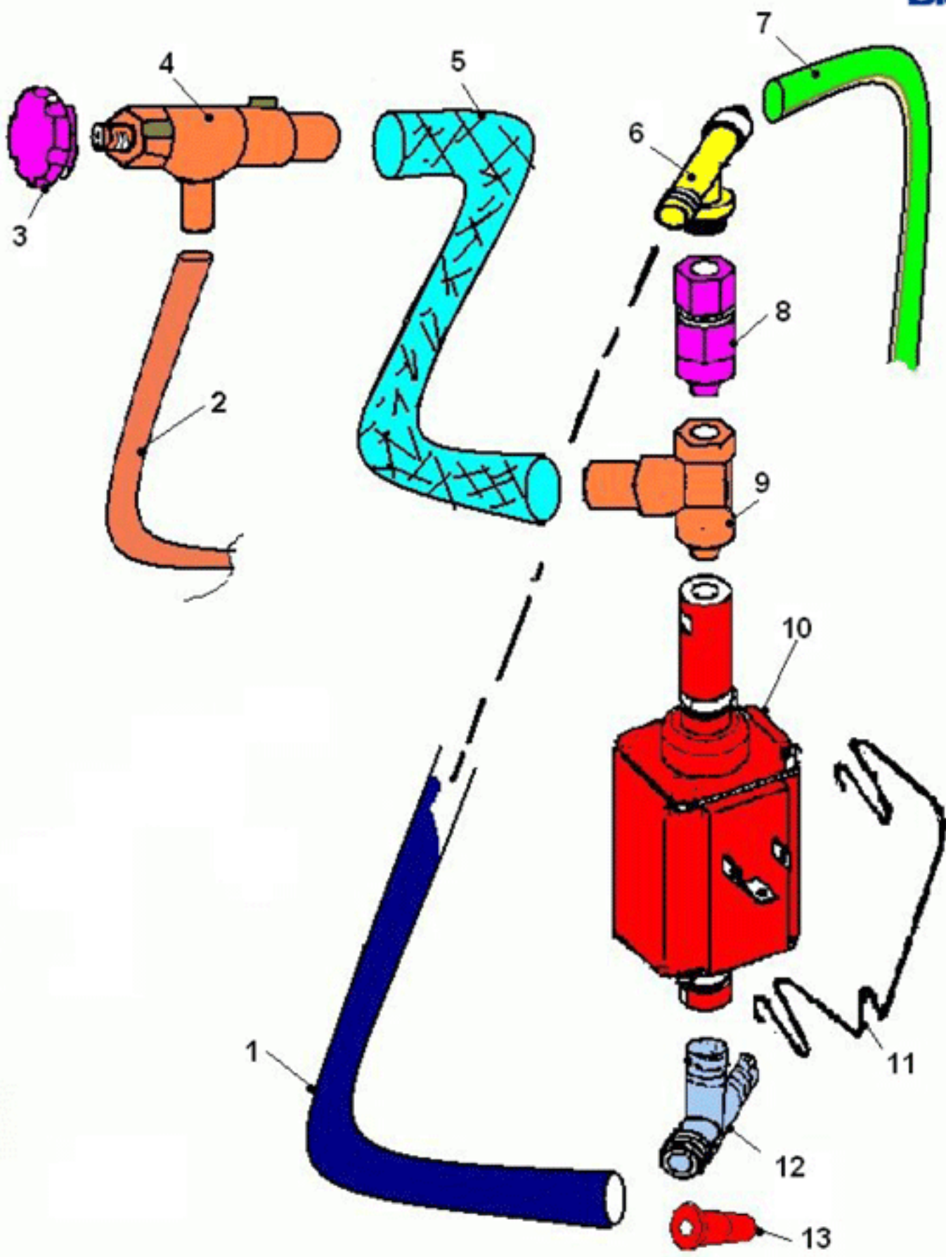
Tavola: ELETTRO-POMPA 220V (565)
