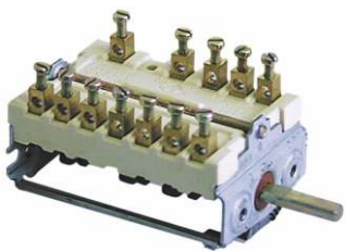
→ kod: 300.081 przełącznik 4-taktowy 16A, mocowanie 6x4,6mm
