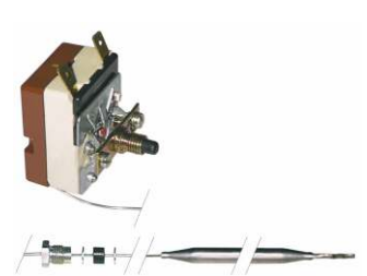
→ kod: 375.138 termostat bezpieczeństwa 230°C, 1-pol., 16A
