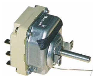
→ kod: 375.097 termostat, t.max. 195°C 95-195°C, 3-pol., 16A
