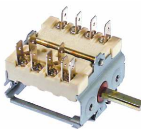
→ kod: 300.166 przełącznik 2-taktowy 16A, mocowanie 6x4,6mm
